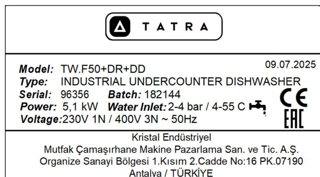
Рисунок 2. TW.F50+DR+DD
