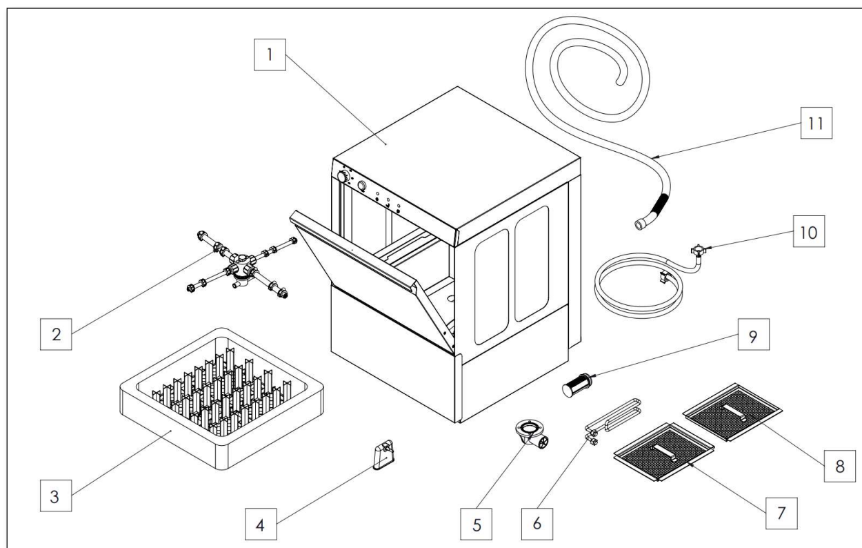
Рисунок 7. TW.F50 Покомпонентное изображение
