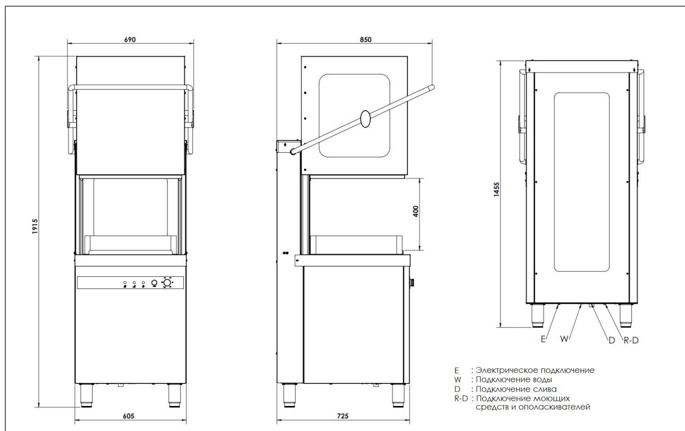
Рисунок 6. TW.H50
