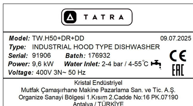
Рисунок 3. TW.H50+DR+DD
