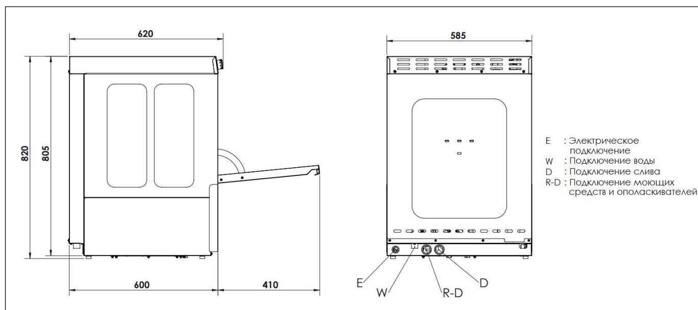
Рисунок 5. TW.F50
