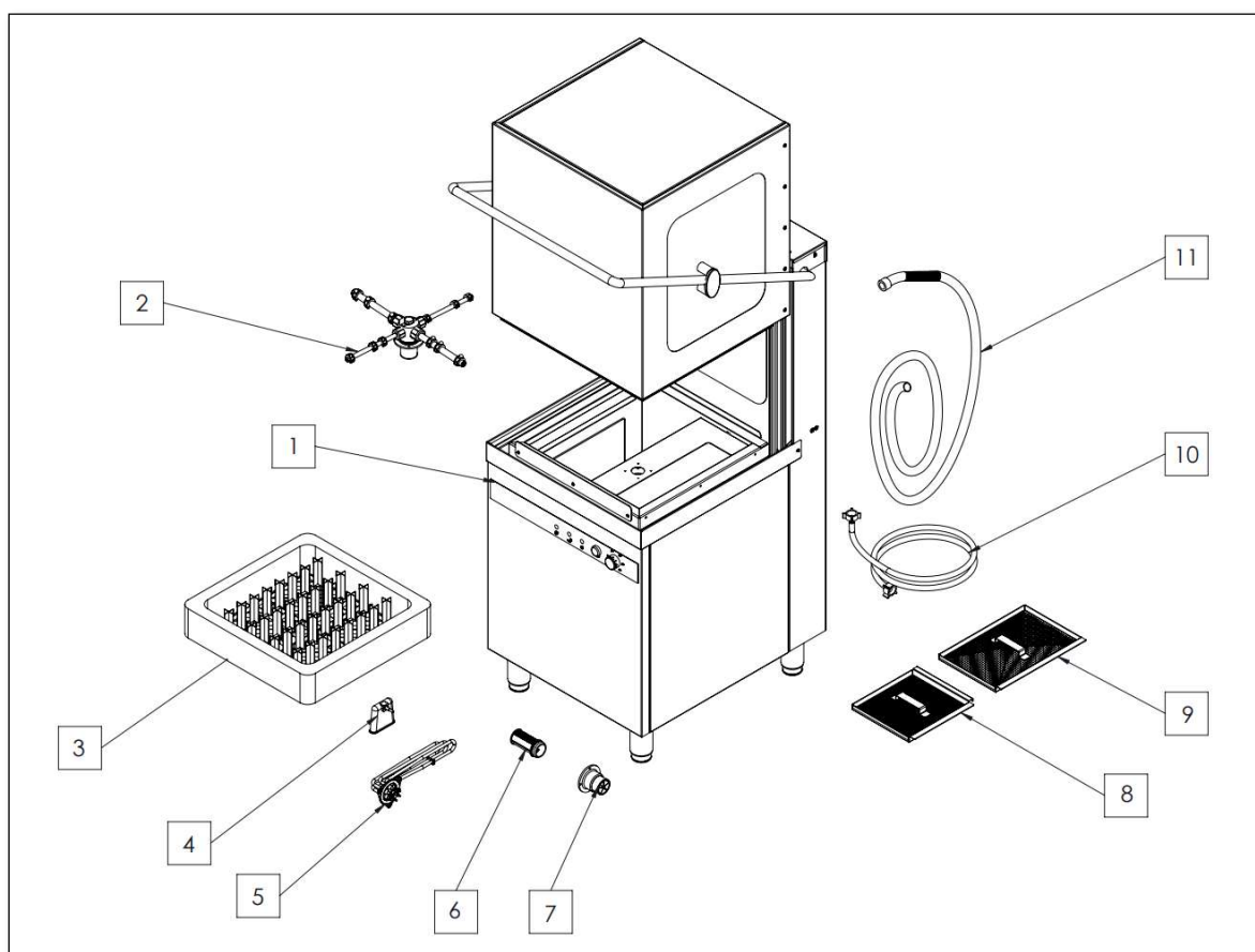
Рисунок 8. TW.H50 Покомпонентное изображение
